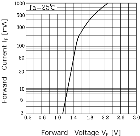
Fig. 1 I_F - V_F
