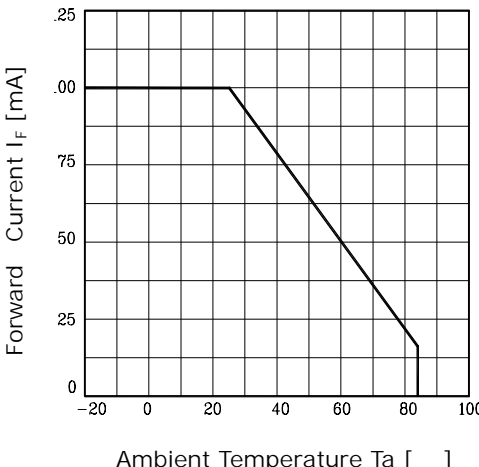
Fig. 3 I_F - T_a
