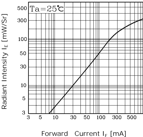
Fig. 2 I_V - I_F
