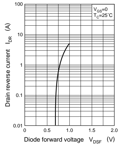
I_{DR} - V_{DSF}
