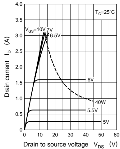
I_D - V_{DS}
