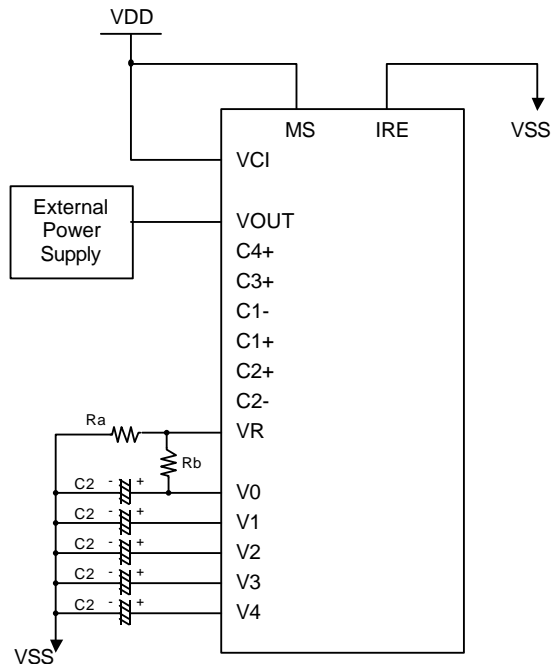
(d) Using external voltage regulator resistors (IRE=0)
