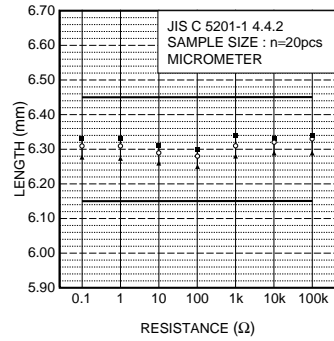
Fig.2 寸法 (長さ)
