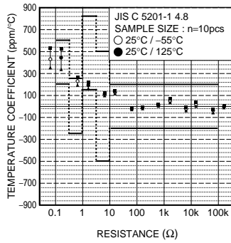
Fig.6 温度による抵抗値変化
