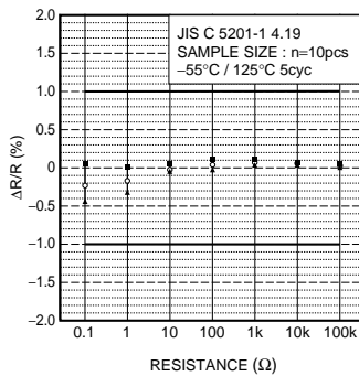
Fig.9 温度急変
