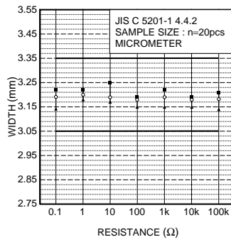
Fig.3 寸法 (幅)
