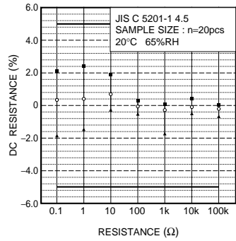
Fig.5 抵抗値
