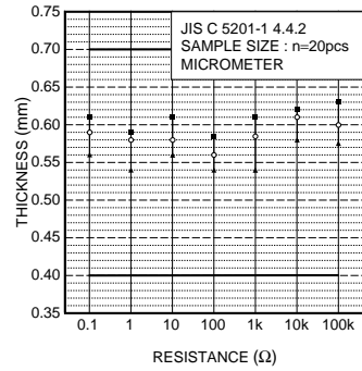
Fig.4 寸法 (厚さ)
