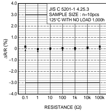
Fig.12 耐久性
