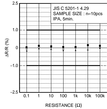
Fig.13 耐溶剤性
