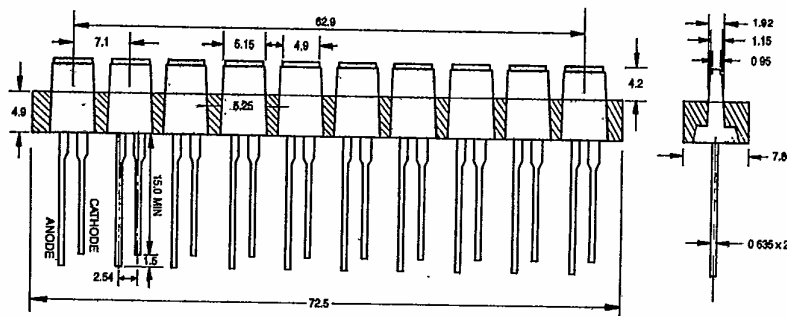
H-5 1x5m/m ARRAY SOCKET 10 SEGUENT
