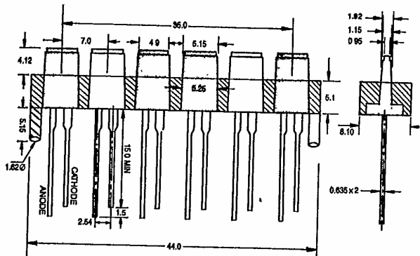
H-1 1x5m/m ARRAY SOCKET 6 SEGUENT
