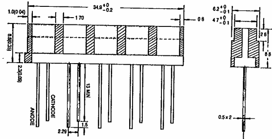
H-2 1.8x5.3m/m ARRAY SOCKET 5 SEGUENT
