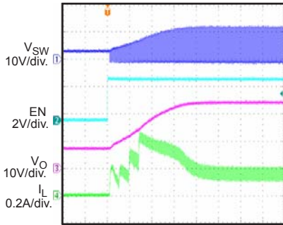
100µs/div
