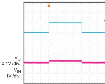
2ms/div
