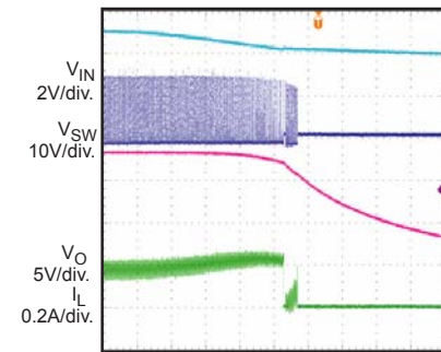
400µs/div
