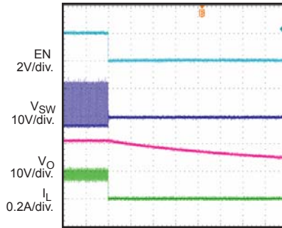
100µs/div
