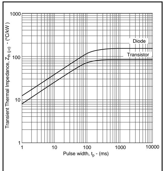
Fig. 11 Transient thermal impedance
