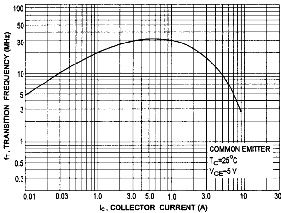
f_T - I_c
