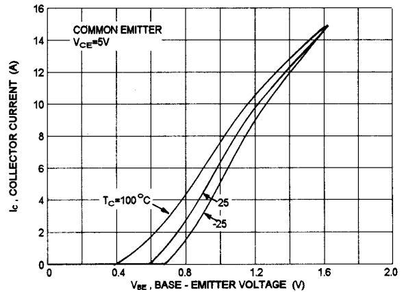
I_c - V_{be}
