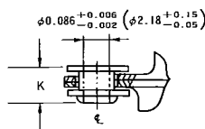
Floating rivet (A-A)
