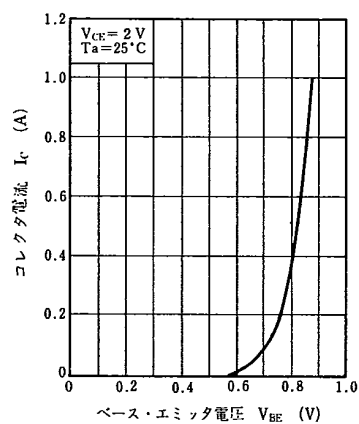
I_C - V_{BE}
