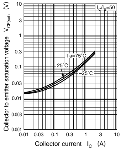
V_{CE(sat)} - I_C
