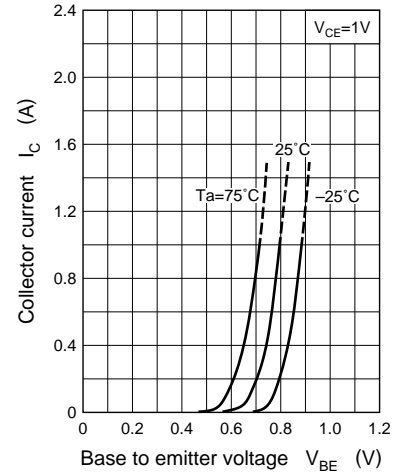
I_C - V_{BE}
