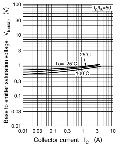
V_{BE(sat)} - I_C
