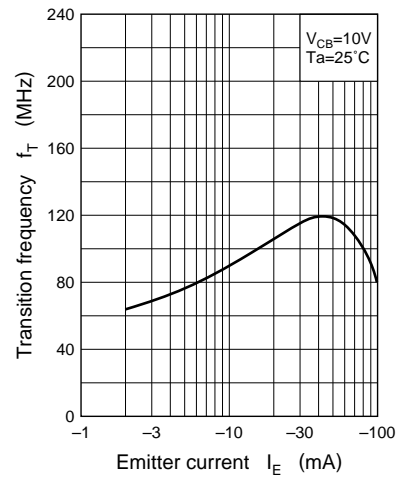
f_T - I_E
