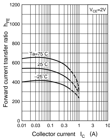
h_{FE} - I_C
