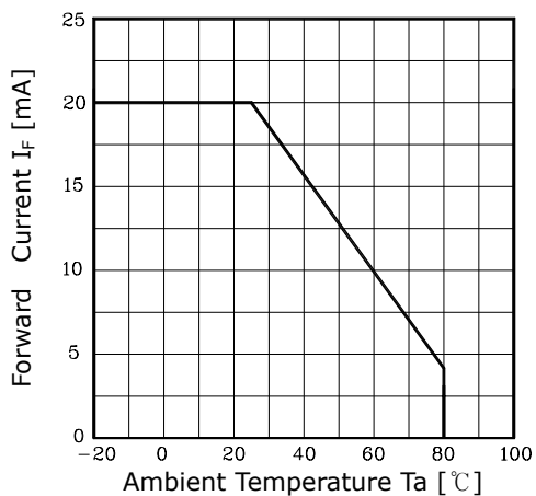
Fig. 3 I_F - T_a
