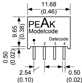
SIP4 – PLASTIC CASE
