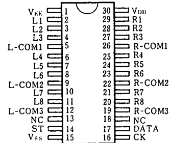
NJU7312AM
