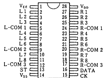
NJU7312AL
