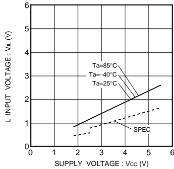
Fig.18 Low input voltage V IL (A0,A1,A2,SCL,SDA,WP)
