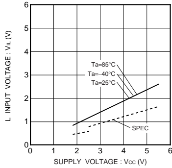
Fig.18 Low input voltage V IL (A1,A2,SCL,SDA,WP)
