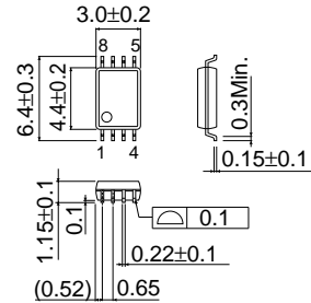
Fig.1(d) PHYSICAL DIMENSION (Units : mm) SSOP-B8 (BR24L01AFV-W)
