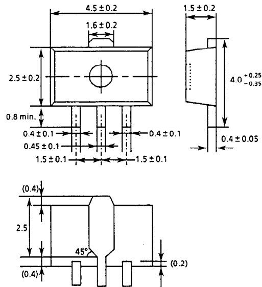
(2) SOT-89-3
