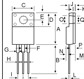
ITO-220AB
