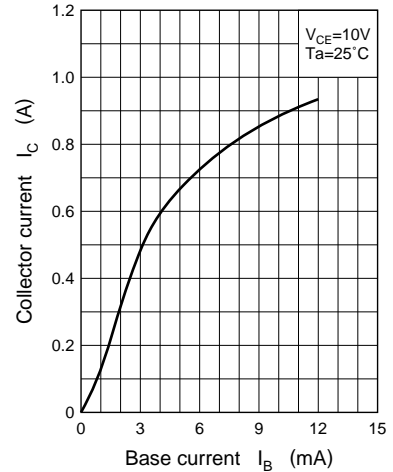
I_C - I_B
