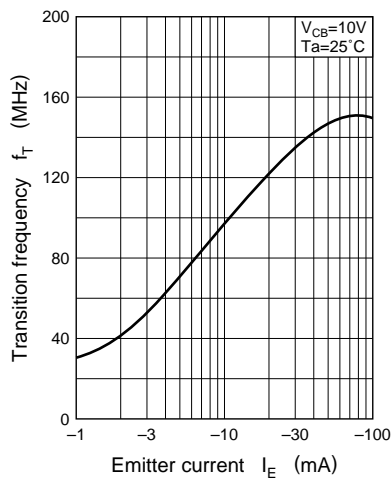
f_T - I_E
