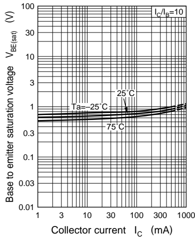
V_{BE(sat)} - I_C
