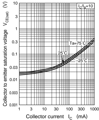
V_{CE(sat)} - I_C
