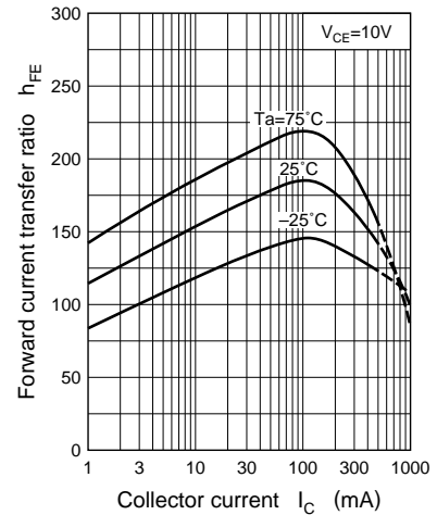
h_{FE} - I_C
