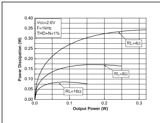
Fig. 23 : Power Dissipation vs Pout
