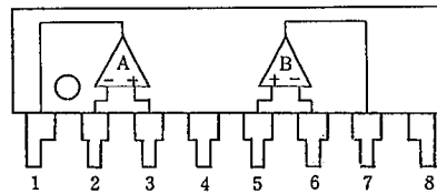
NJM5532L
