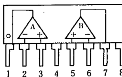
NJM4560L
