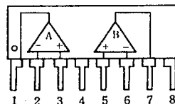
NJM062L
