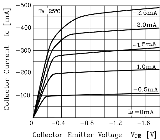
Fig. 3 I_C - V_{CE}
