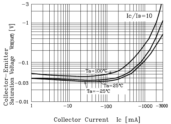
Fig. 4 V_{CE(sat)} - I_C
