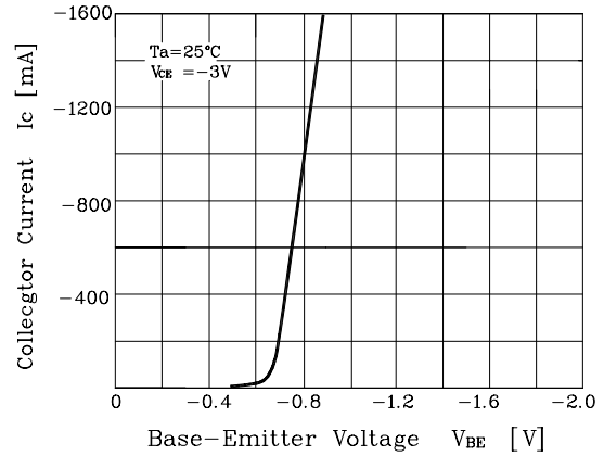
Fig. 2 I_C - V_{BE}
