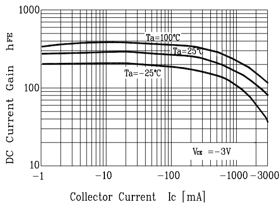
Fig. 5 h_{FE} - I_C
