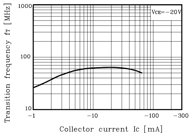
Fig. 3 f_T - I_C
