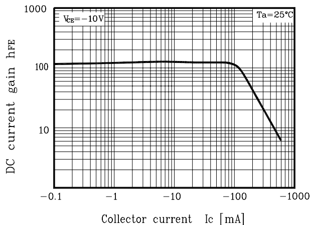
Fig. 1 h_{FE} - I_C
