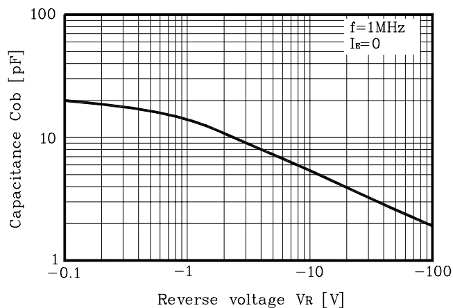
Fig. 4 C_{ob} - V_R
