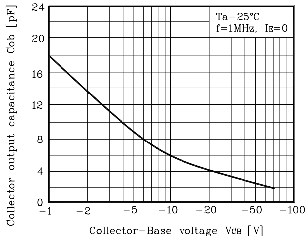
Fig. 5 C_{ob} - V_{CB}
