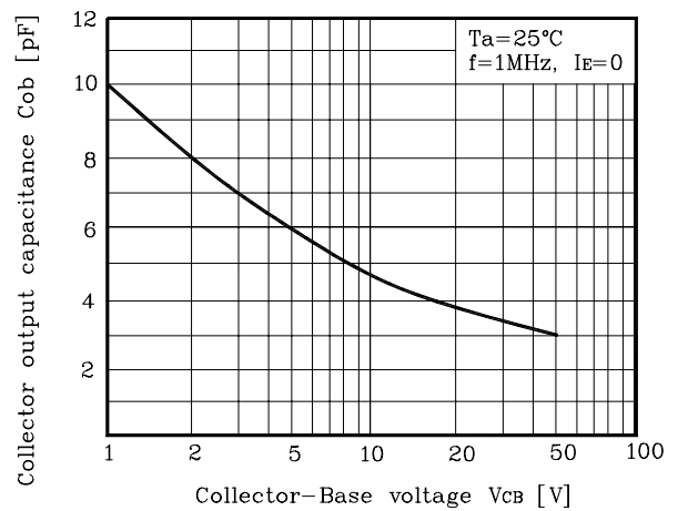
Fig. 4 C_{ob}-V_{CB}
