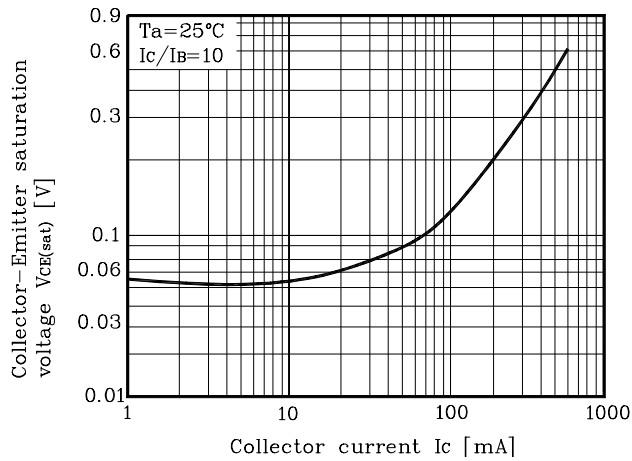
Fig. 3 V_{CE(sat)}-I_C
