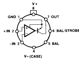
TO-99 (J-Suffix)
