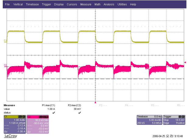
SFS5-5 53mV
