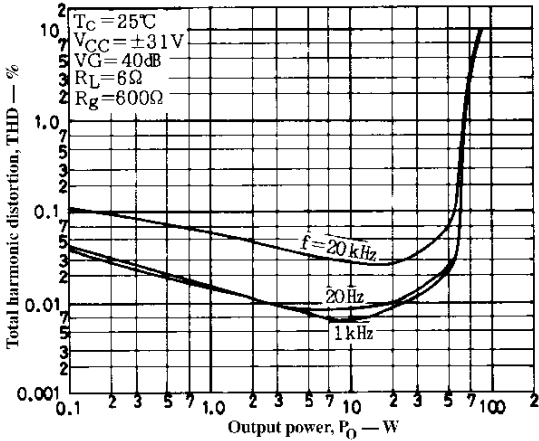
THD - P_O
