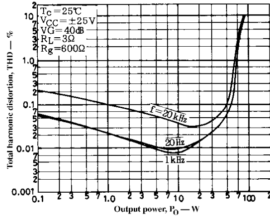
THD - P_O
