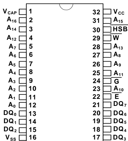
32 Pin SOIC
