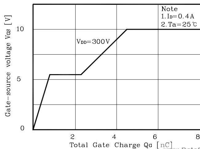
Fig. 6 V_{GS} - Q_G
