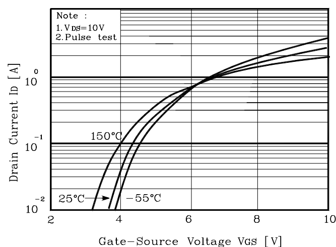
Fig. 2 I_D - V_{GS}
