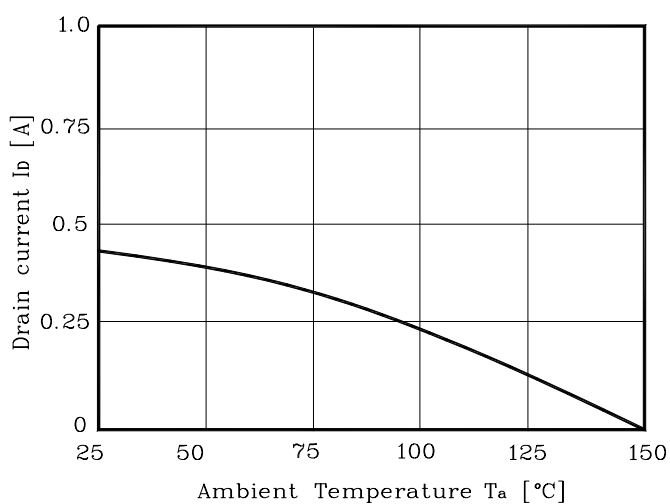
Fig. 9 I_D - T_a
