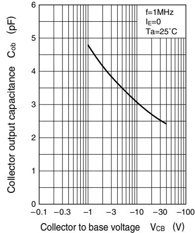
C_{ob} - V_{CB}
