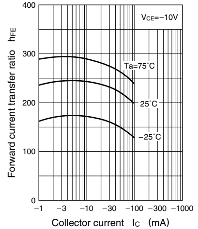
h_{FE} - I_C
