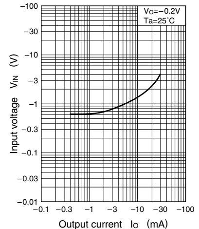
V_{IN} - I_O
