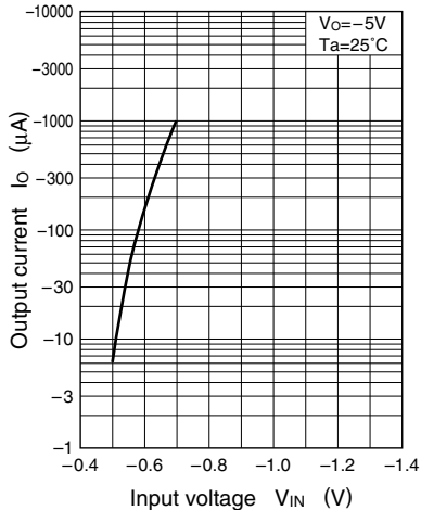
I_O - V_{IN}
