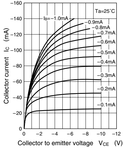
I_C - V_{CE}
