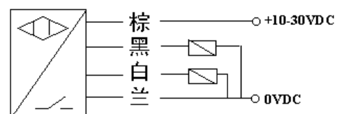
图4: PNP常开和常闭四线输出
