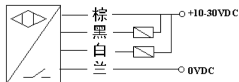
图3: NPN常开和常闭四线输出
