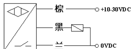
图2: PNP常开或常闭三线输出
