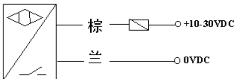
图5: 直流二线输出
