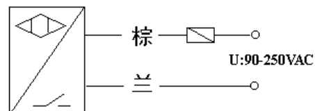
图6: 交流二线输出
