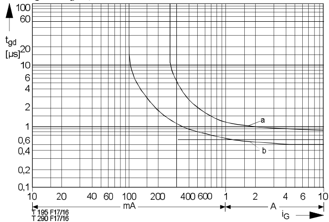
Bild / Fig. 16 Zündverzögerung/Gate controlled delay time t_{gd} . DIN 41787, t_a = 1 \mu s , t_j = 25^\circ C . a - äußerster Verlauf/limiting characteristic b - typischer Verlauf/typical characteristic
