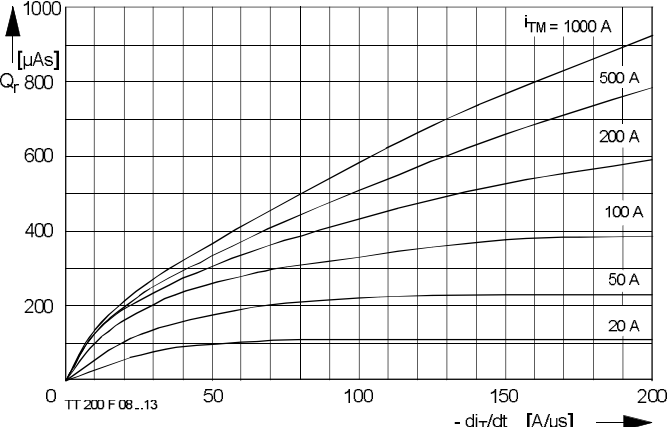
Bild / Fig. 17 Sperrverzögerungsladung Q_r = f(di/dt) t_j = t_{j \max} , v_R = 0.5 V_{RRM} , v_{RM} = 0.8 V_{RRM} Parameter: Durchlaufstrom I_{TM} Recover charge Q_r = f(di/dt) t_j = t_{j \max} , v_R = 0.5 V_{RRM} , v_{RM} = 0.8 V_{RRM} Parameter: on-state current I_{TM}
