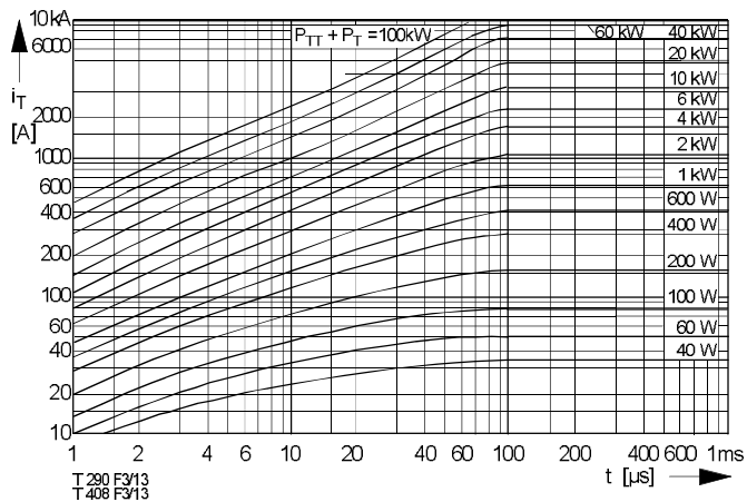
Bild / Fig. 13 Diagramm zur Ermittlung der Summe aus Einschalt- und Durchlaufverlustleistung ( P_{TT} + P_T ) je Zweig. Diagram for the determination of the sum of the turn-on and on-state power loss per arm ( P_{TT} + P_T ).
