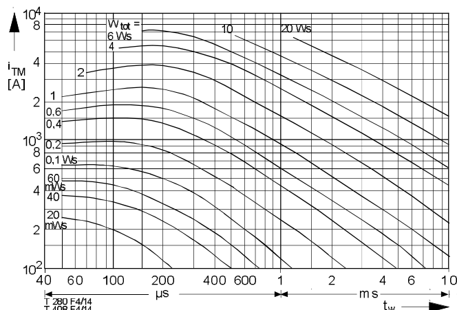
Bild / Fig. 14 Diagramm zur Ermittlung der Gesamtenergie W_{tot} für einen sinusförmigen Durchlauf-Strompuls für einen Zweig. Diagram for the determination of the total energy W_{tot} for a sinusoidal on-state current pulse for one arm.
