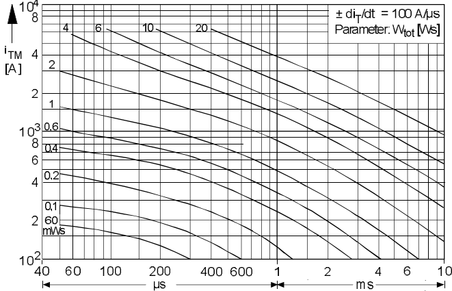
Bild / Fig. 7, 8, 9 Diagramme zur Ermittlung der Gesamtenergie W_{tot} für einen trapezförmigen Durchlaß-Strompuls, für einen Zweig bei: der angegebenen Stromsteilheit di_T/dt , Vorwärts-Sperrspannung V_{DM} \leq 0,67 V_{DRM} , Rückwärts-Sperrspannung V_{RM} \leq 50V , Spannungssteilheit dv_R/dt \leq 100 V/\mu s .
