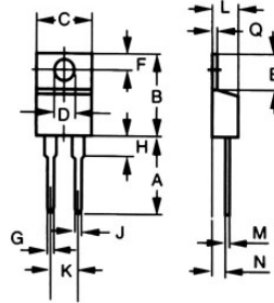
Dimensions TO-220AC
