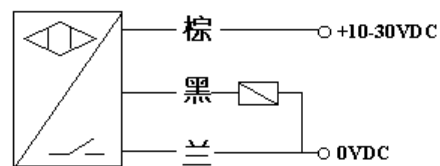
图2: PNP常开或常闭三线输出
