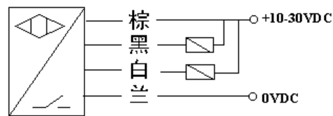
图3: NPN常开和常闭四线输出
