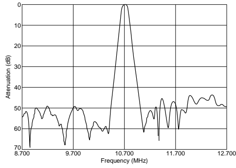
SFECV10M7KA00-R0
