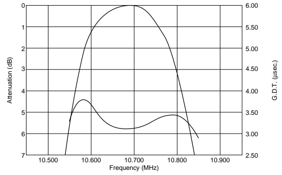
SFELA10M7GA0G-B0
