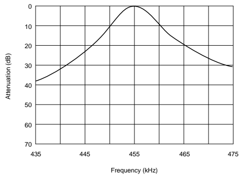
IFT+PFSLA455KP2A-B0
