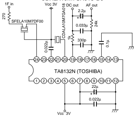
CDALA10M7GA018-B0
