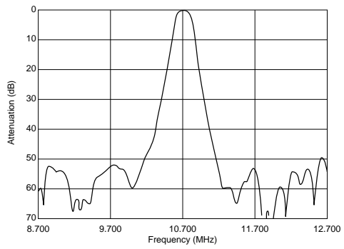
SFELB10M7GA00-B0
