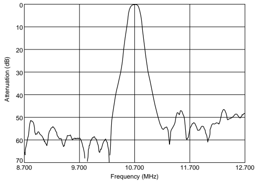
SFECV10M7HA00-R0
