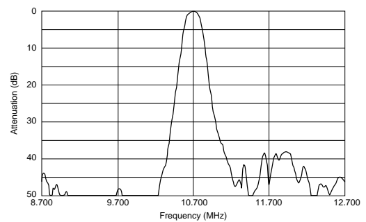
SFECS10M7GA00-R0
