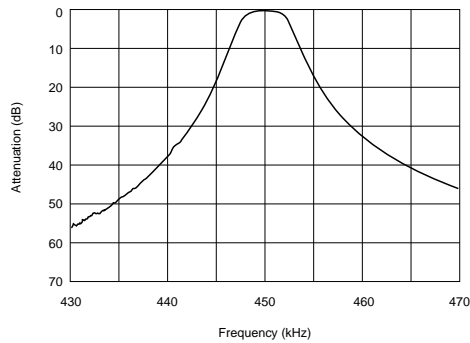
IFT+PFWCC450KS2A-R0
