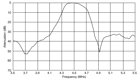
SFSRA4M50DF00-B0
