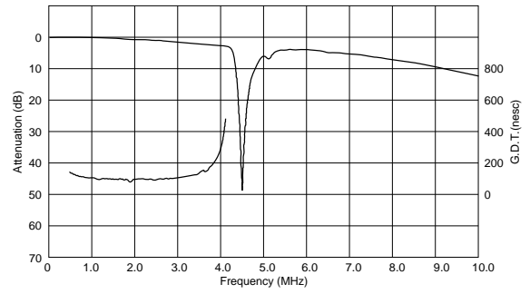
TPSRA4M50C00-B0
