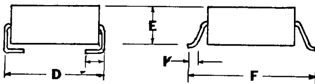
DO-214AA
