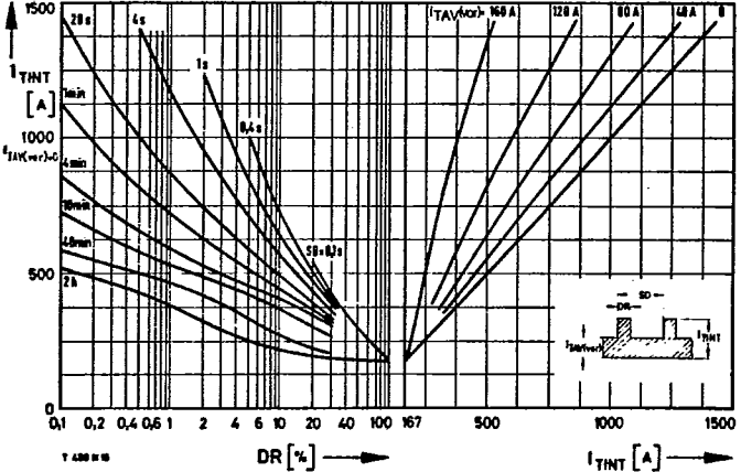
Bild/Fig. 16 Höchstzulässiger Durchlaßstrom I_{TINT} bei Aussetzbetrieb und beidseitiger Luftselbstkühlung, t_A = 45^{\circ}C , Kühlkörper K0.36S. Limiting on-state current I_{TINT} during intermittent operation at natural two-sided cooling, t_A = 45^{\circ}C , heatsink type K0.36S. Parameter: Spieldauer/cycle duration SD Vorlaststrom/pre-load current I_{TAV(vor)}
