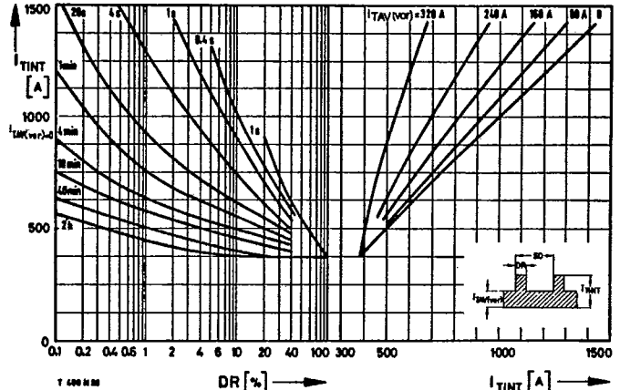
Bild/Fig. 17 Höchstzulässiger Durchlaßstrom I_{TINT} bei Aussetzbetrieb und verstärkter beidseitiger Luftkühlung, t_A = 35^{\circ}C , Kühlkörper K0.12F, V_L = 50 l/s. Limiting on-state current I_{TINT} during intermittent operation at forced two-sided cooling, t_A = 35^{\circ}C , heatsink type K0.12F, V_L = 50 l/s. Parameter: Spieldauer/cycle duration SD Vorlaststrom/pre-load current I_{TAV(vor)}
