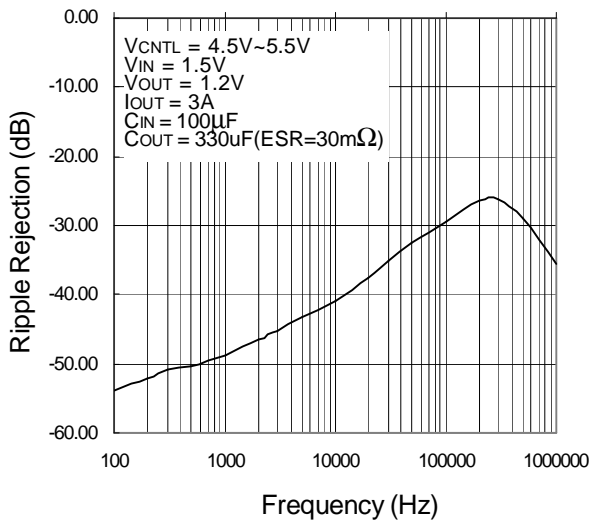
VCNTL PSRR
