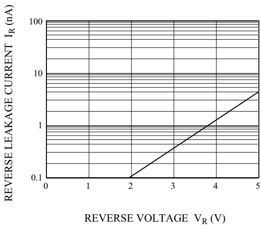
Fig. 3 I_R - V_R
