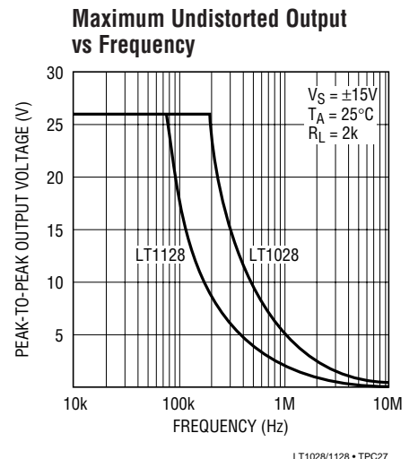
LT1028/1128 • TPC27
