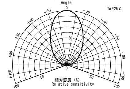
■ 指向特性
