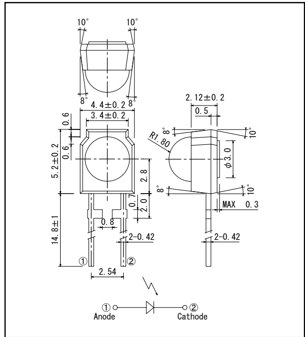
※アクティブエリア 1.70×1.70(mm)
