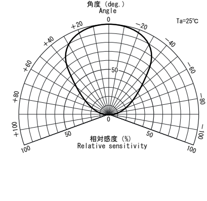
■指向特性
