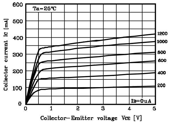
Fig. 4 I_C - V_{CE}
