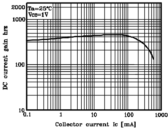
Fig. 3 h_{FE} - I_C
